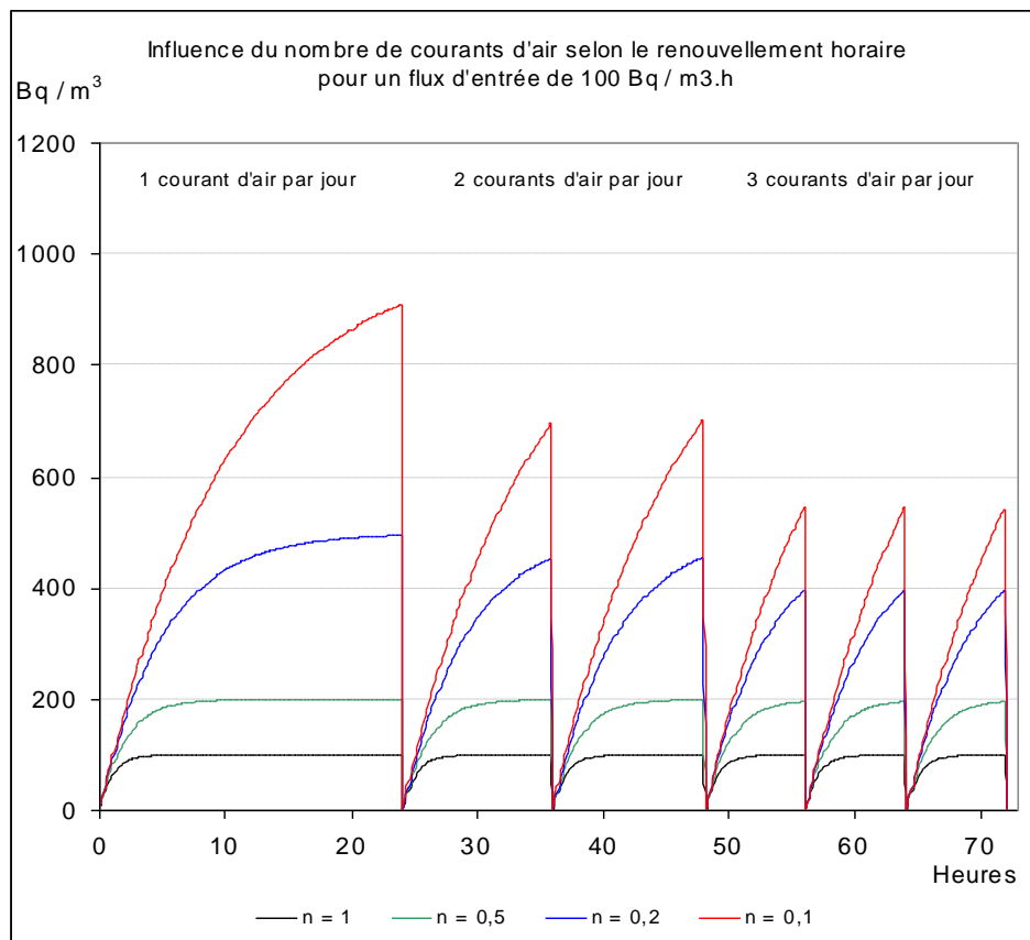
FIGURE A4. ACTIVITÉ VOLUMIQUE DU RADON DANS UN LOCAL EN FONCTION DU NOMBRE DE COURANTS D'AIR JOURNALIER ET DU RENOUELEMENT D'AIR HORAIRE.
