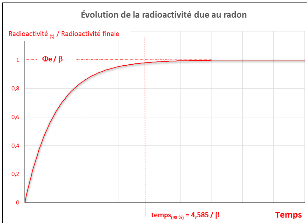
FIGURE A2. ÉVOLUTION TYPIQUE DE LA RADIOACTIVITÉ DUE AU RADON 222 POUR UN FLUX D'ENTRÉE ET UNE AÉRATION CONSTANTS.
