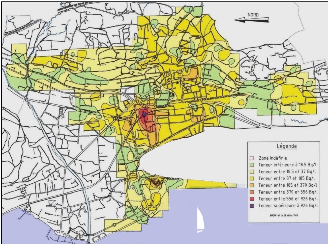
FIGURE 3. LE RADON DANS LE SOL d'AIX-LES-BAINS.
